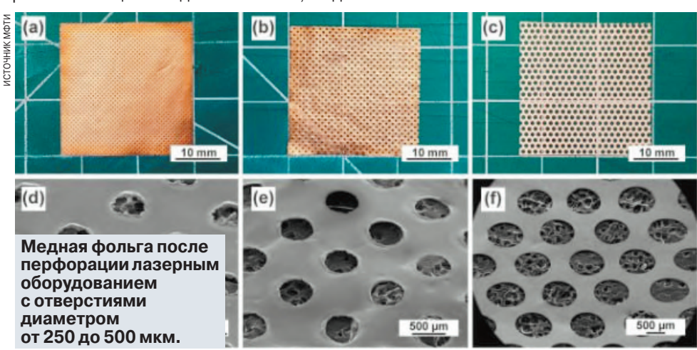
Медная фольга после перфорации лазерным оборудованием с отверстиями диаметром от 250 до 500 мкм.
