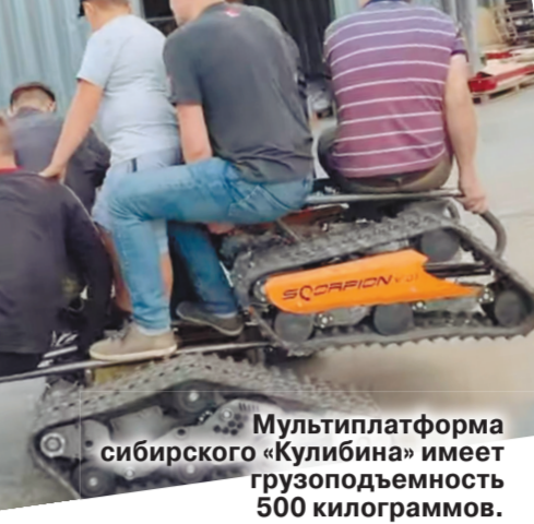
Мультиплатформа сибирского «Кулибина» имеет грузоподъемность 500 килограммов.
