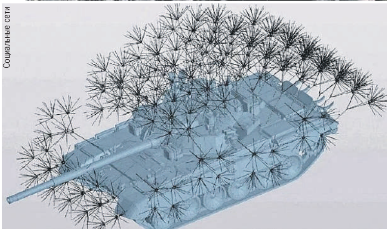
Вот так на схеме и в жизни выглядит танк, защищенный «одуванчиками» из стеклопластика.
