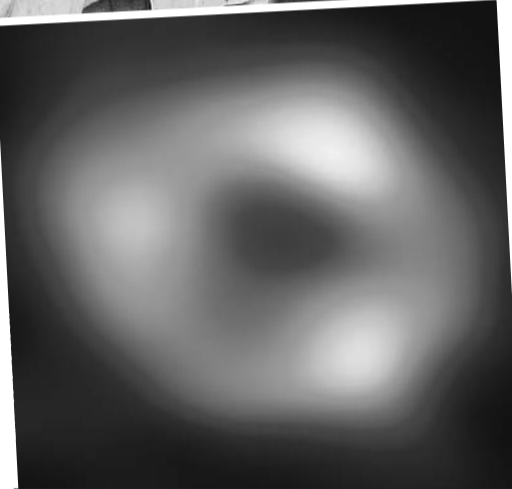
На фотографии мы видим «тень» черной дыры в центре и светящееся вещество вокруг нее в виде бублика.
