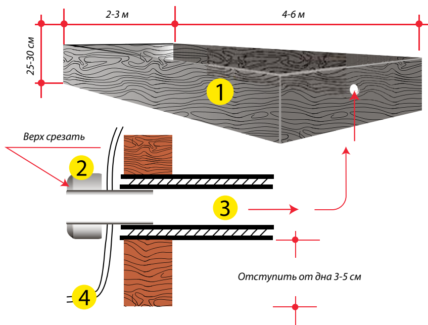
СХЕМА АВТОСЛИВА
